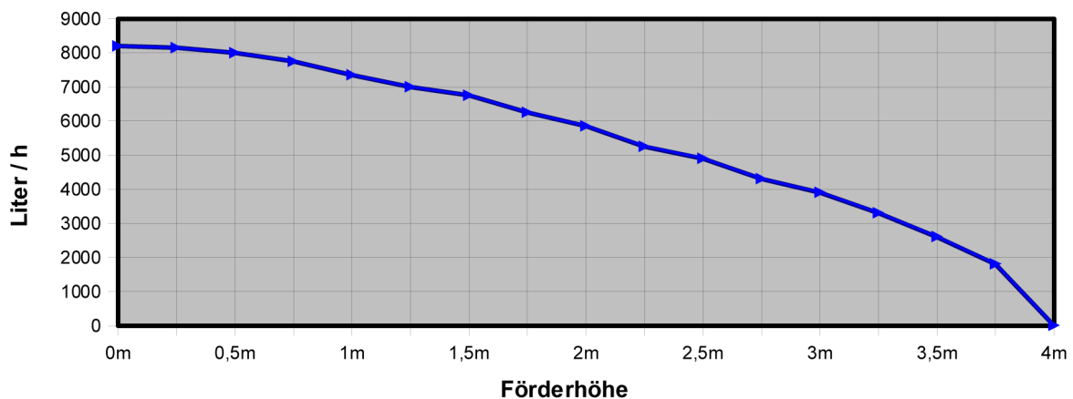
Leistungsdiagramm
