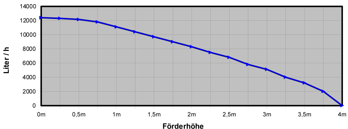
Leistungsdiagramm
